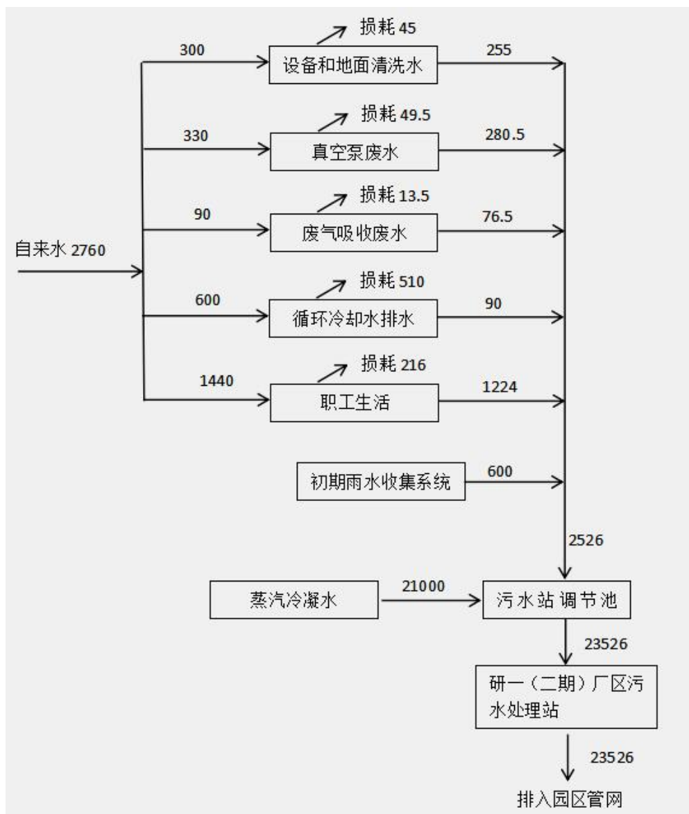
图3-4 项目水平衡图 单位 (t/a)
