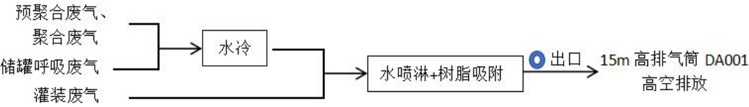
图 7-2 有组织废气监测点位图
