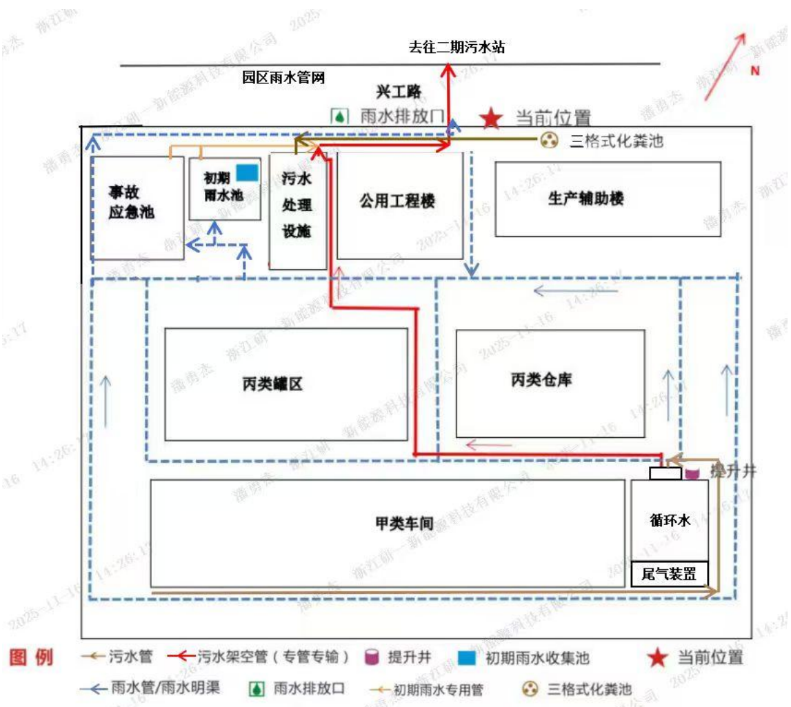
图3-3 项目平面布置图
