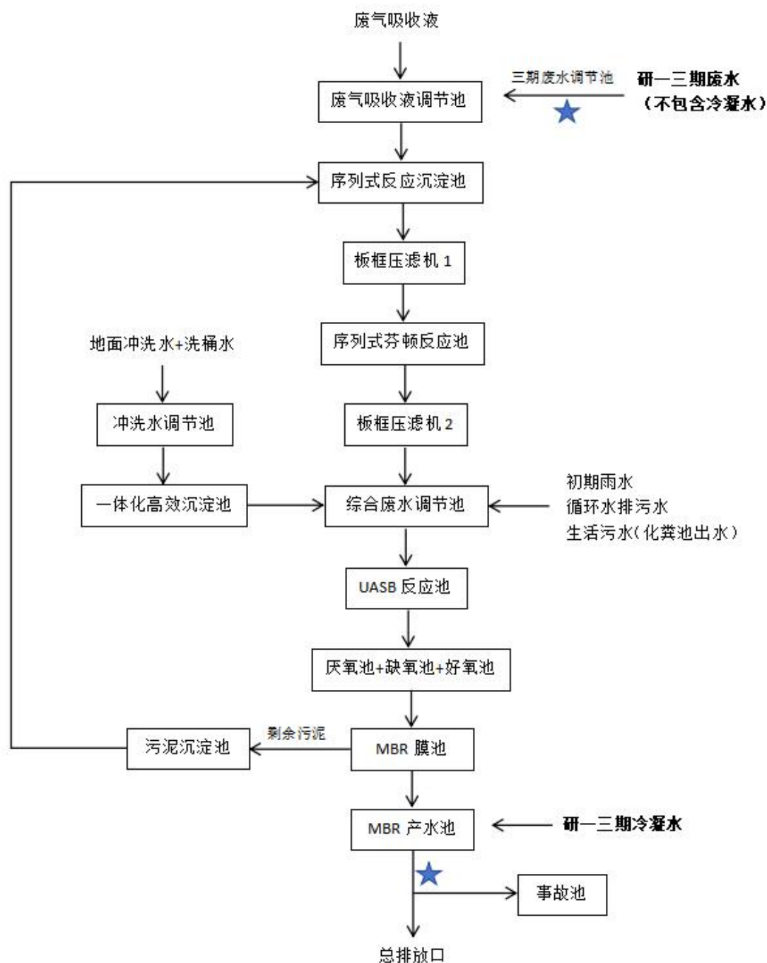
图4-1 本项目污水处理工艺图
