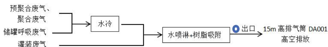
图4-2 废气处理设施工艺流程图
